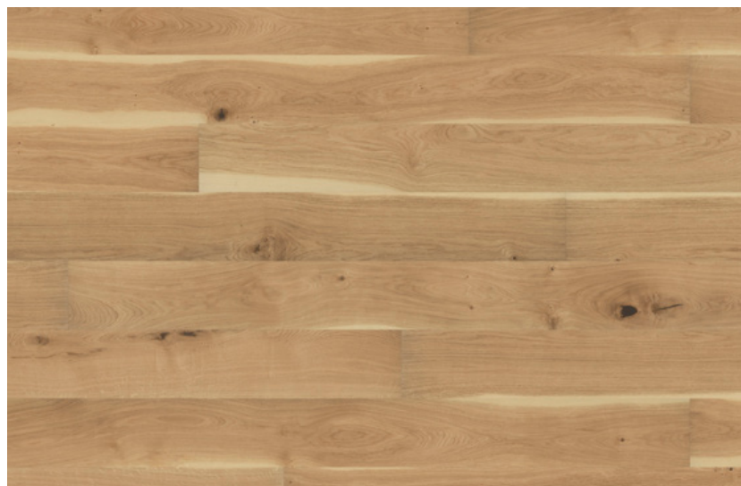
⑧ No. 115.15 Eiche Rohholzoptik Naturöl 2420 x 187 x 13 mm 4-seitig gefast, gebürstet, mit Splint
