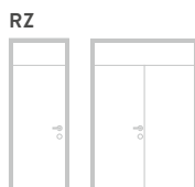
Raumhohe Zarge mit Querteil mit Kämpfer bis Stocklichthöhe von 2.520 mm (einflügelig, zweiflügelig)
